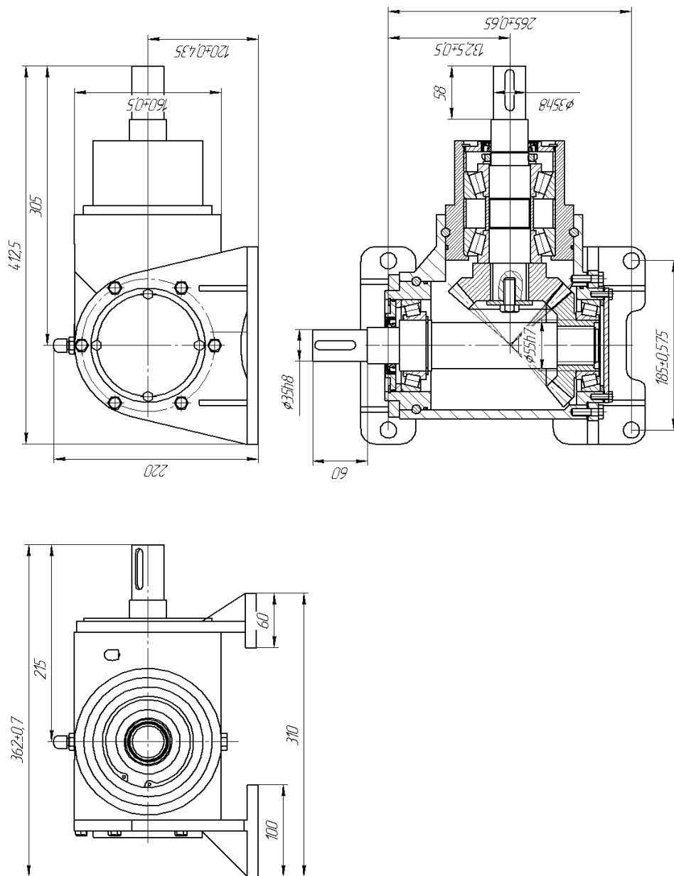
Рисунок 1 –Присоединительные размеры редуктора
